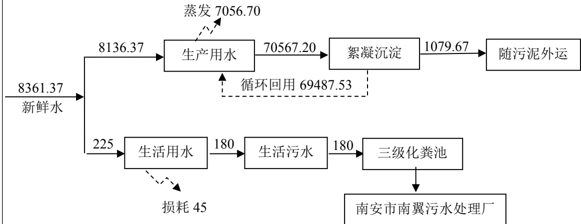
图 2-1 项目给排水平衡图 (单位: t/a)
